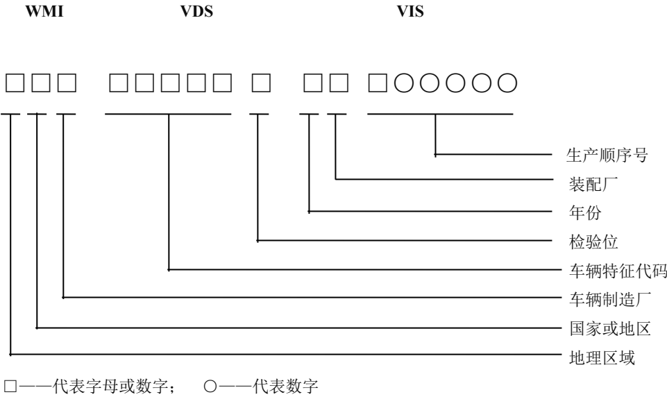
图1 年产量大于等于 1000 辆的完整车辆和/或非完整车辆制造厂车辆识别代号结构示意图
